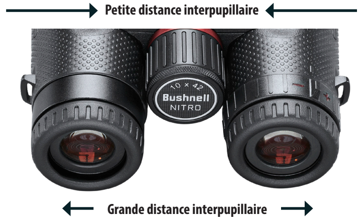
Fig. 3 Inter-pupillaire Ajustement de la distance
